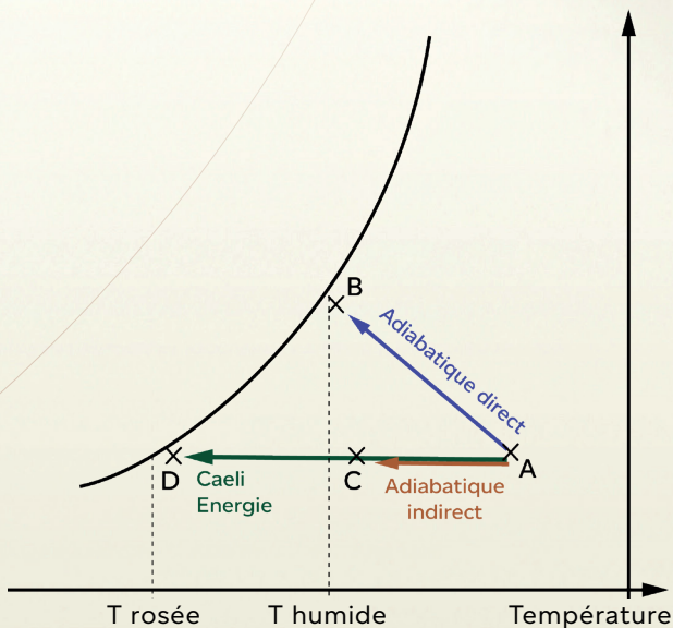
→ FIGURE 1 : PERFORMANCES DES SYSTÈMES DE RAFFRAÎCHISSEMENT ADIABATIQUE
